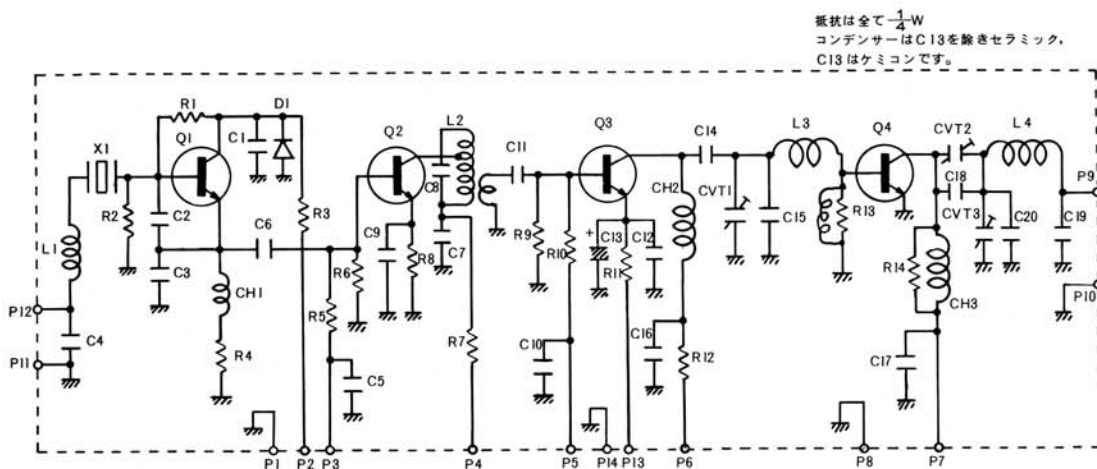
図-2 回路図
