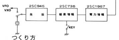
図-1 ブロック図
