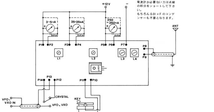
図-7 基板のピン接続図
