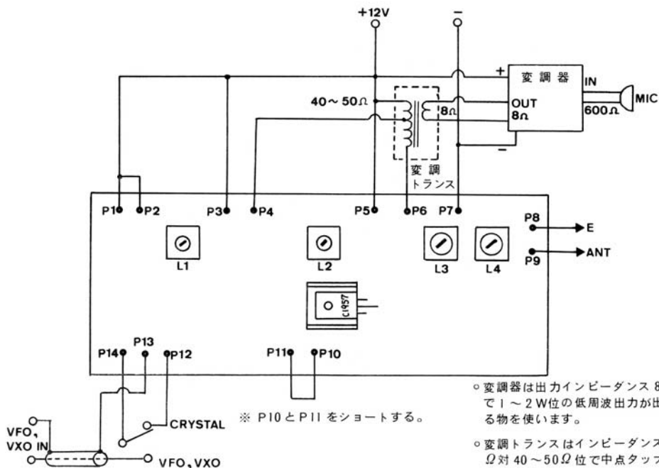
図-13 AM変調のかけ方
