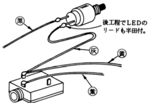
3.5 φステレオジャック （KEY ジャック）
