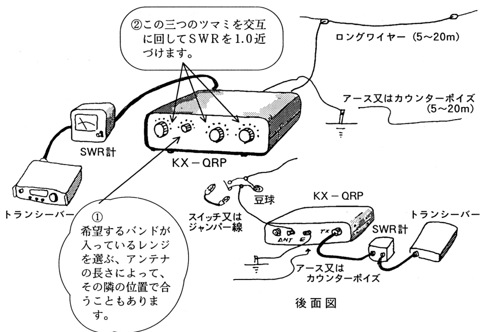
第3図 接続のようすと調整手順
