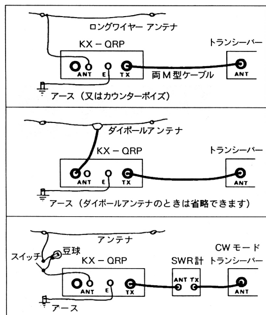
第2図 各アンテナとの接続図
