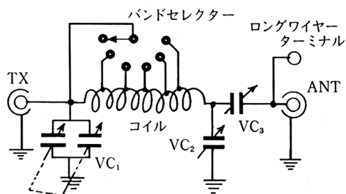
第1図 回路図
